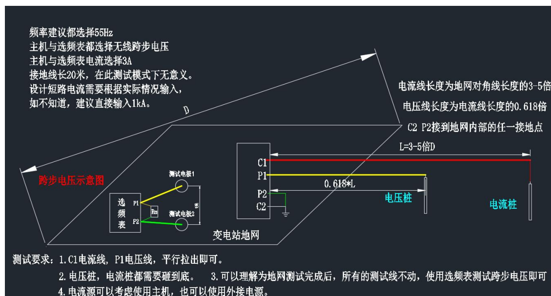
图53 无线跨步电压测量接线图
