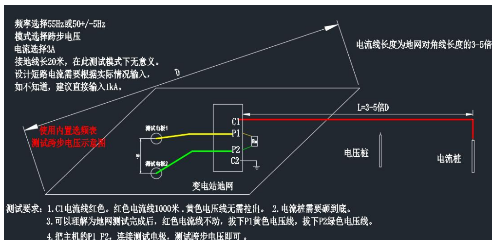
图55 使用内置选频表测试跨步电压接线图
