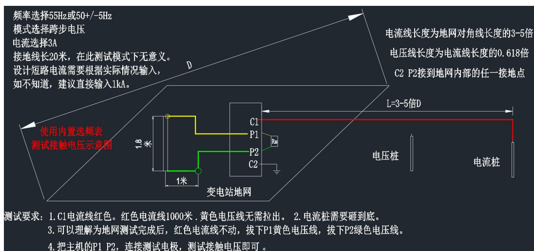
图56 使用内置选频表测试接触电压接线图
