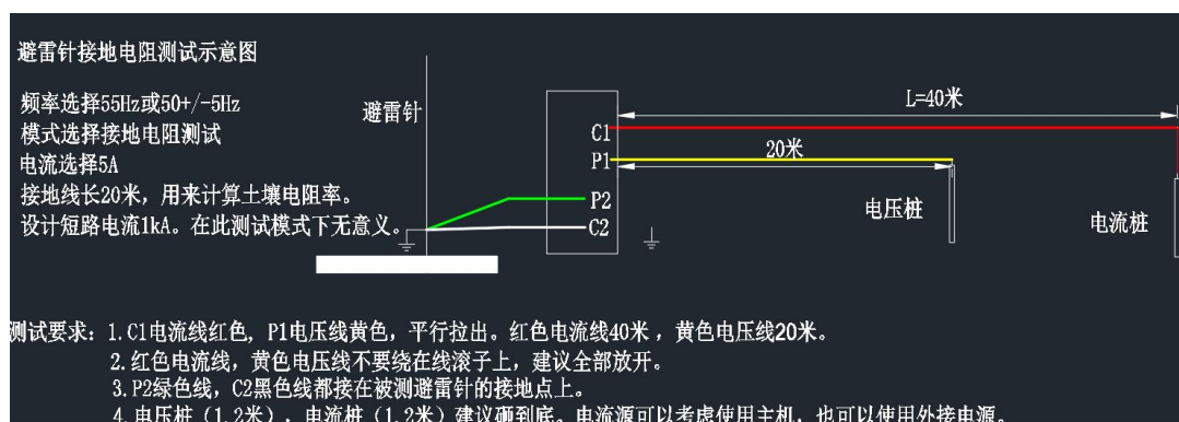
图52 避雷针接地电阻测量接线图
