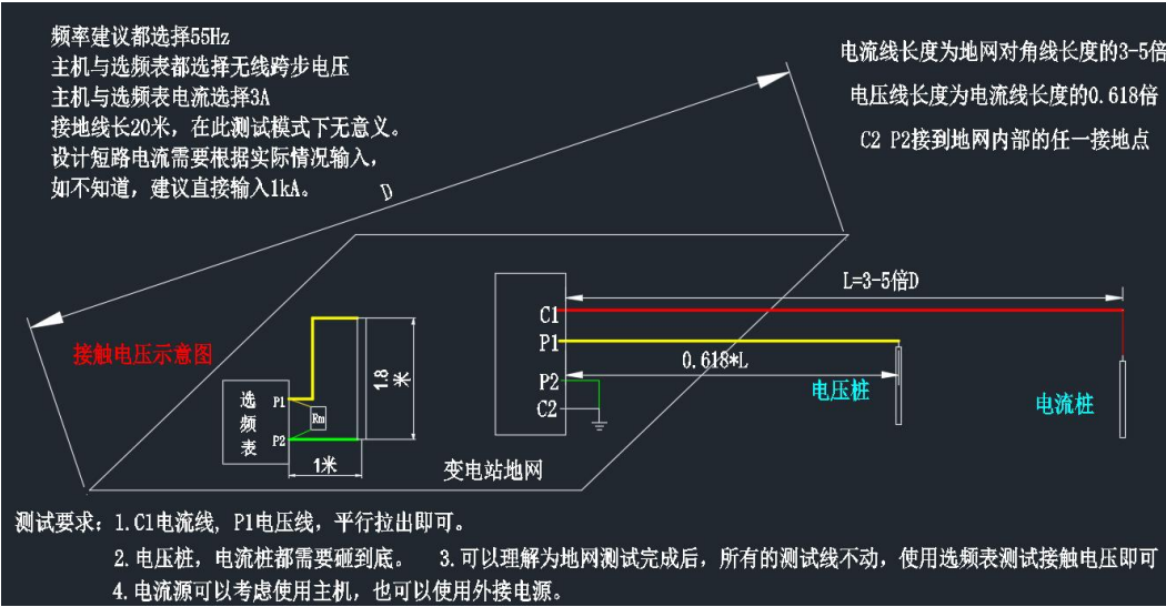
图54 无线接触电压测量接线图
