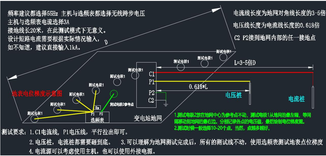
图54 无线地表点位梯度测量接线图
