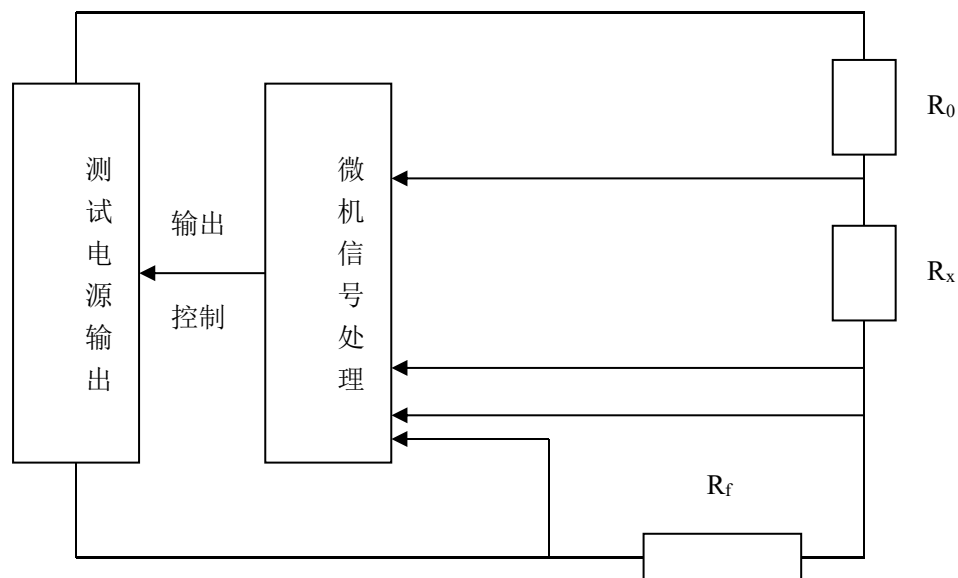
图 1 测量原理示意图
