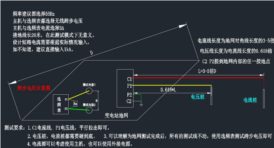
跨步电压测量接线图
