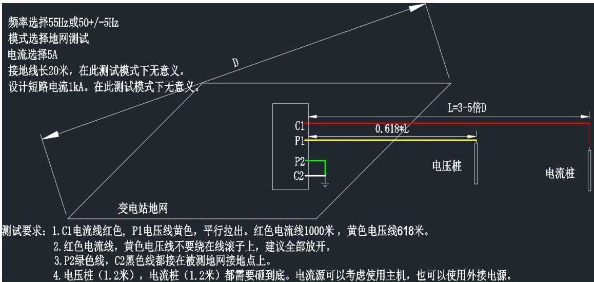
图50 夹角法测试地网阻抗测量接线图
