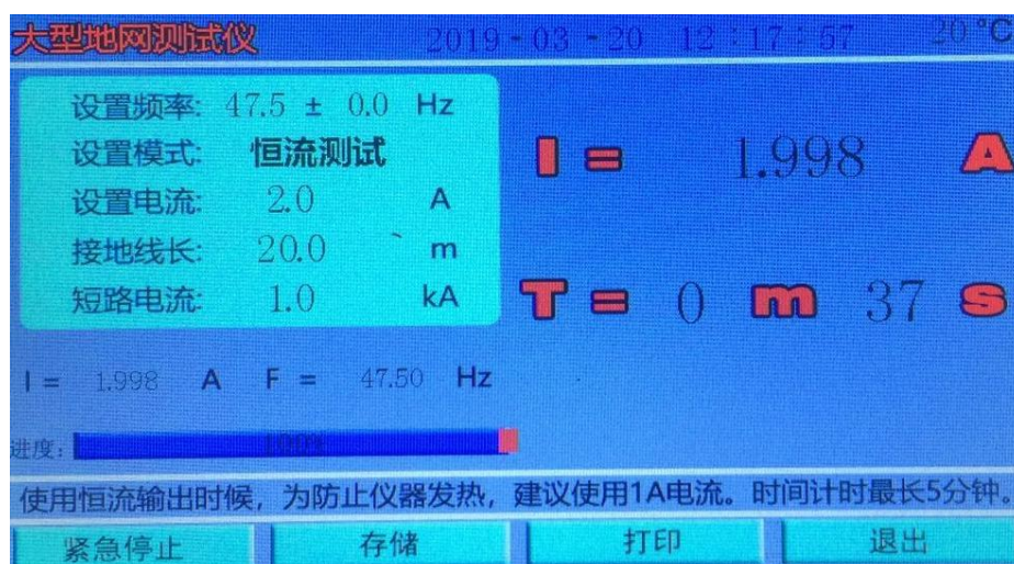
图 20 恒流测试结果界面
