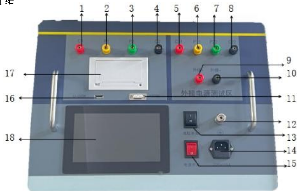
图 2 面板示意图
