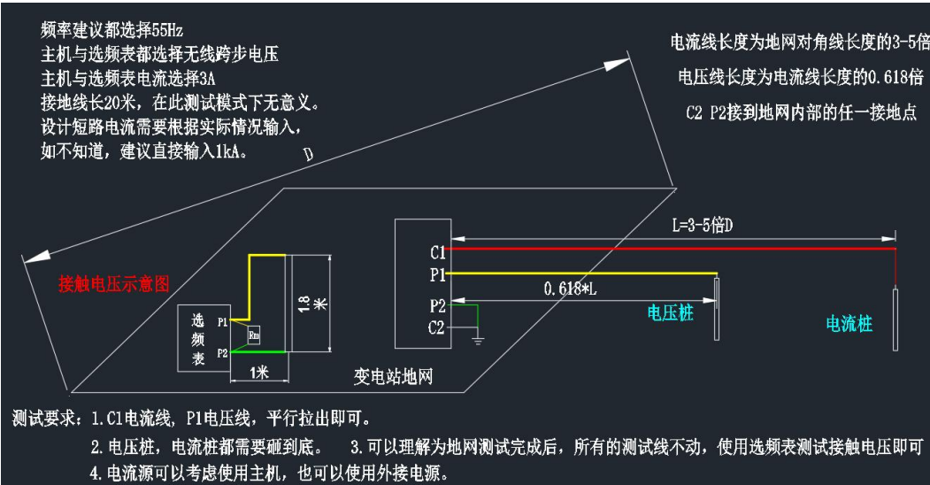
接触电压测量接线图
